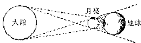
日食
