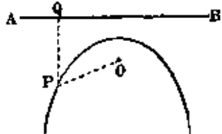
抛物线
