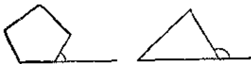
外角①
