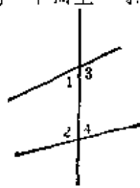
内错角
