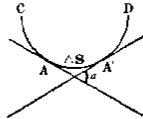
曲率
