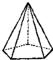
棱锥
