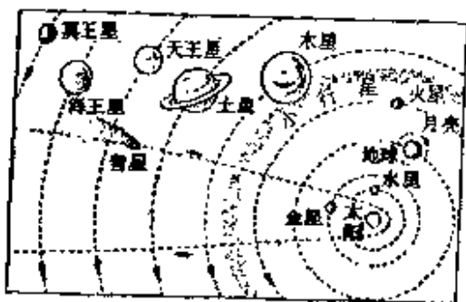
太阳系
