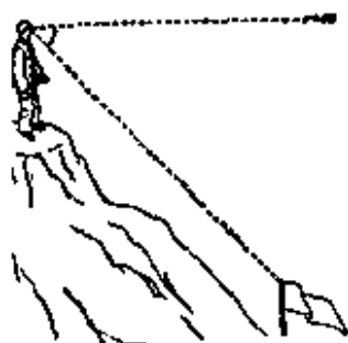
钩角 俯角
