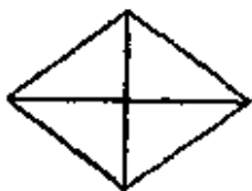
菱形
