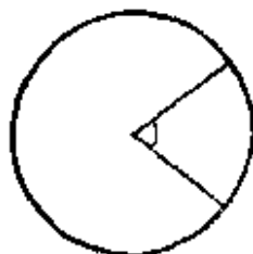
圆心角
