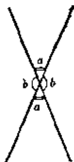
对 顶 角
