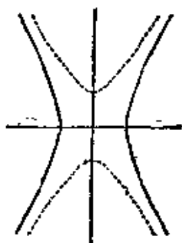
双曲线
