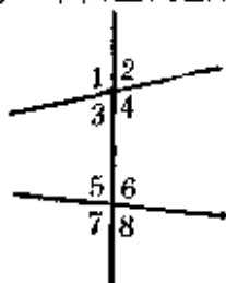
同位角
