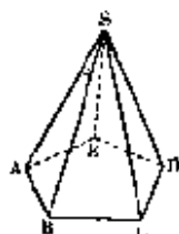
多 面 角
