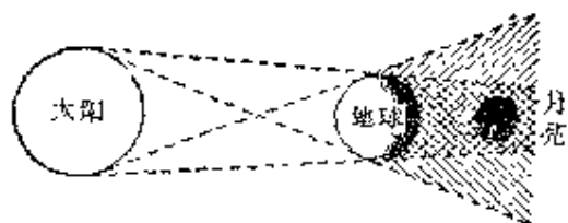
月食
