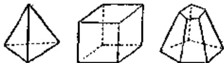
多面体
