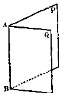
二 面 角
