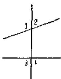
外错角
