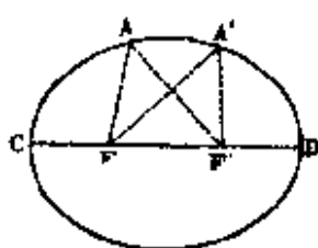
椭圆
