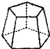
棱锥台
