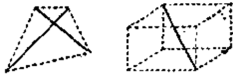
对角线
