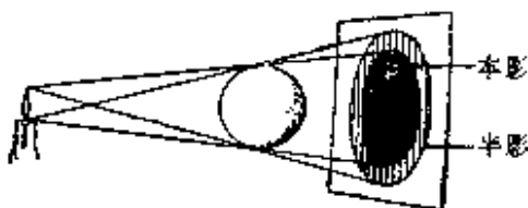
本影和半影
