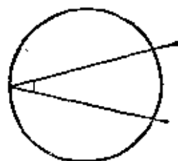
圆周角
