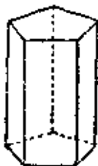
棱柱体
