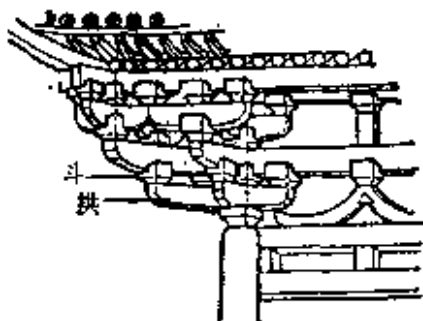
斗 拱
