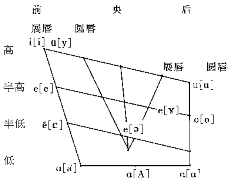
舌面元音舌位图
